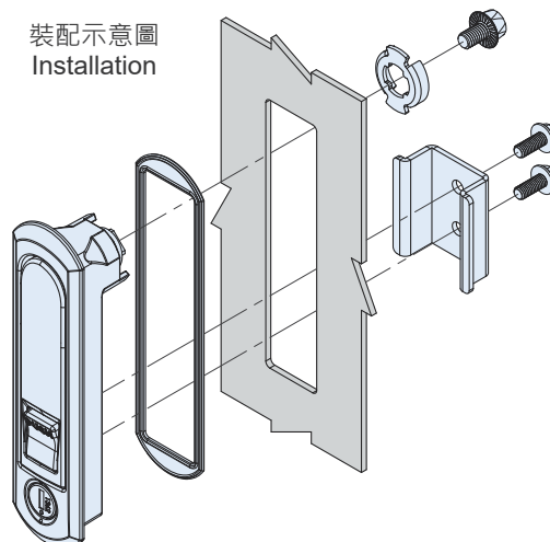
左開多點連桿裝配示意圖 Installation
