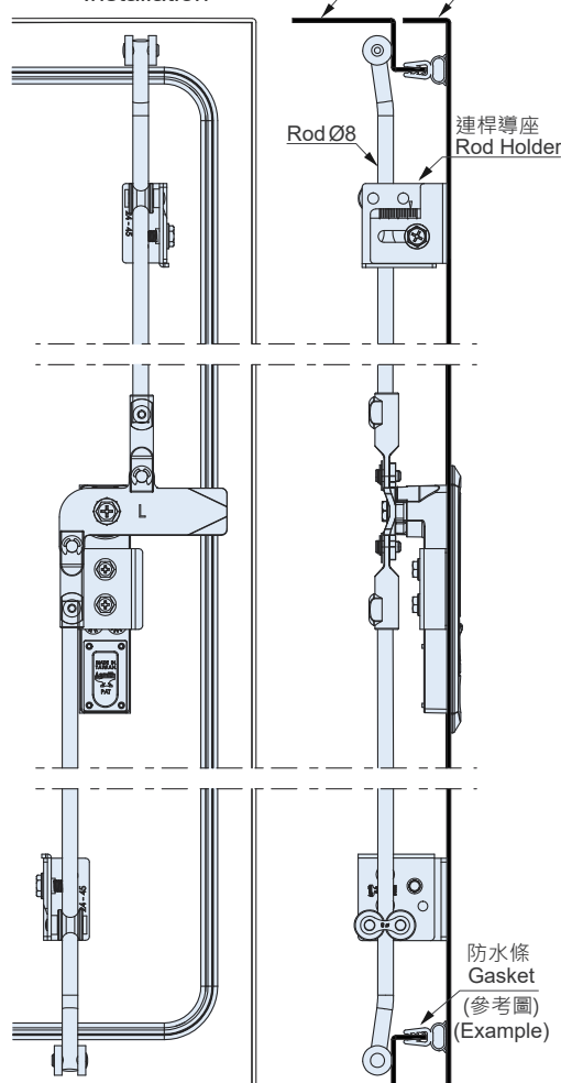
左開多點連桿裝配示意圖 Installation
