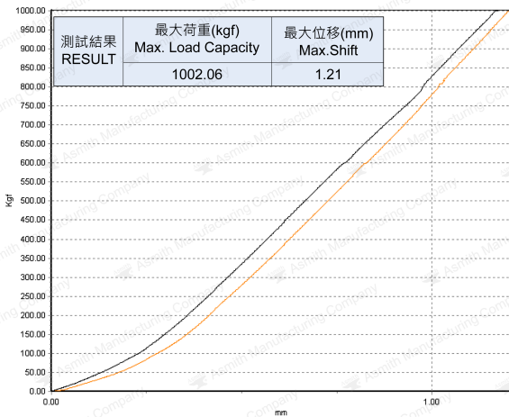
M8主體下壓測驗
