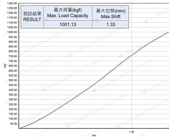
M16主體下壓測驗
