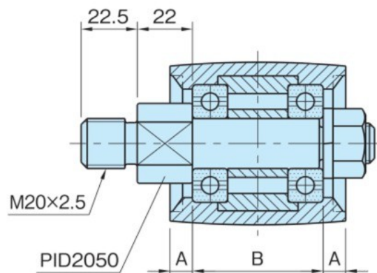
CTR 6065 (樹脂製)
