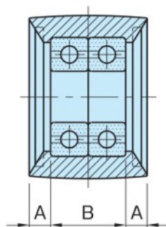
CTR 3050~5560 (樹脂製)
