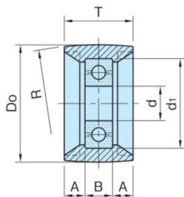
CTR 1535~2550 (樹脂製)
