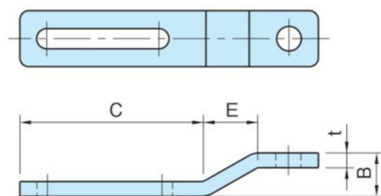
CRT (クランク タイトナー)
