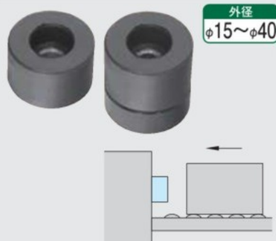
フィクスト ダンパー
