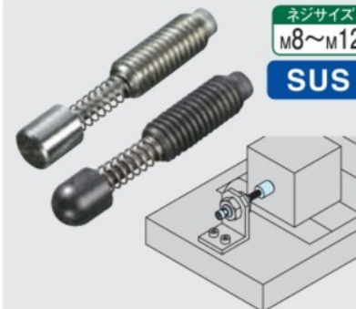
スプリング突き出しピン
