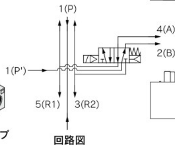
回路図
