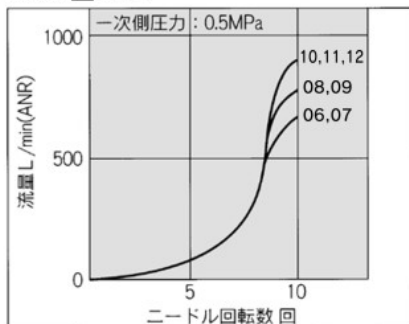
AS32□1FG AS33□1FG
