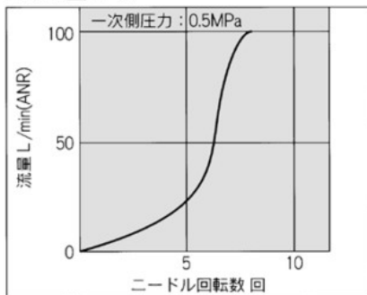
AS32□1FG AS33□1FG
