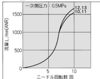
AS42□1FG AS43□1FG
