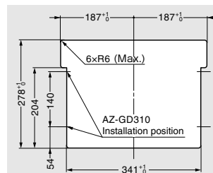
AZ-GD310-HL AZ-GD310-BL
