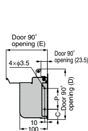
AZ-GD180-HL
