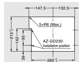
AZ-GD230-HL AZ-GD230-BL
