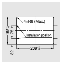
AZ-GD180-HL
